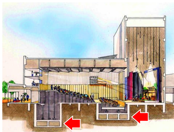
多目的ホール断面図 矢印の部分が地下ピット
