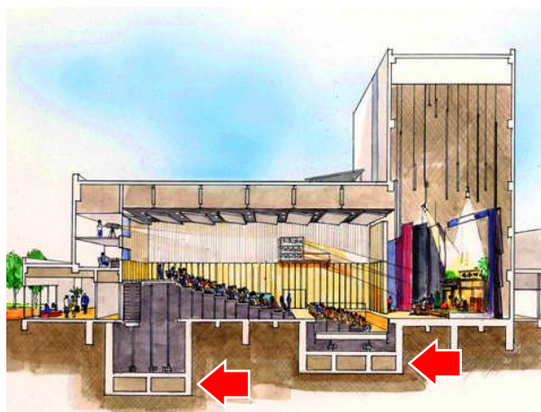
多目的ホール断面図 矢印の部分が地下ピット
